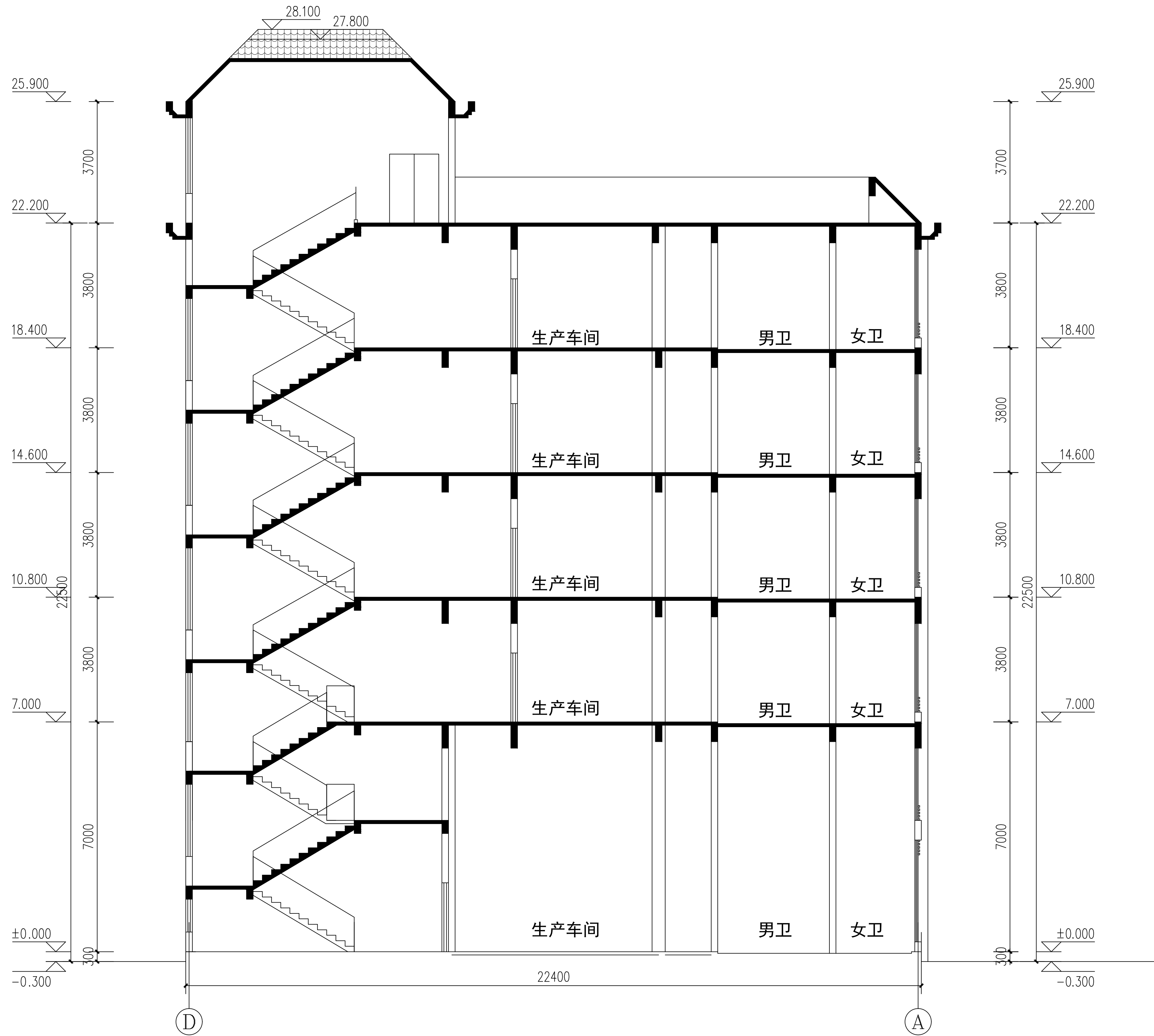
3#厂房1-1剖面图 1:100
