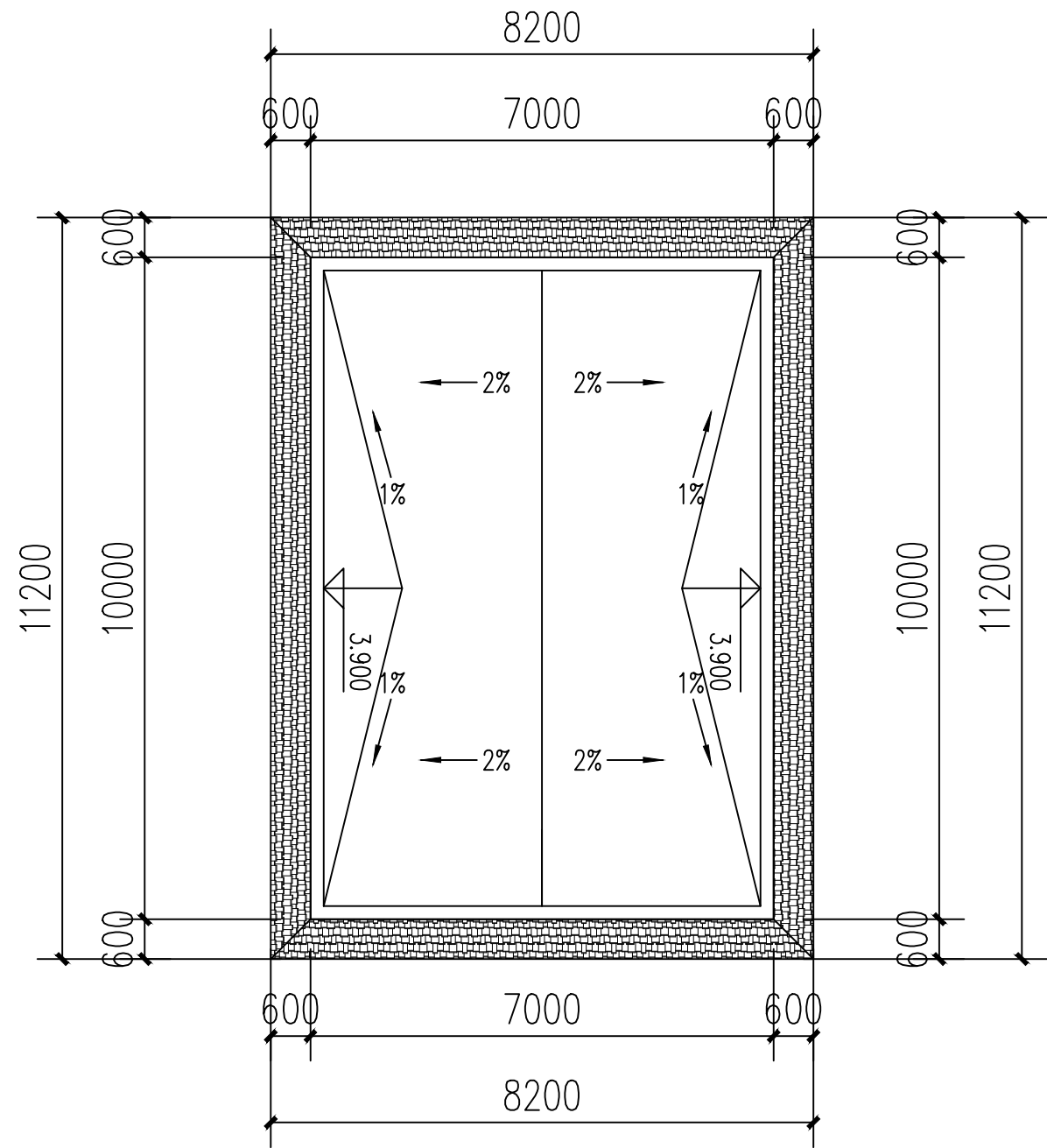
水池泵房屋顶平面图
