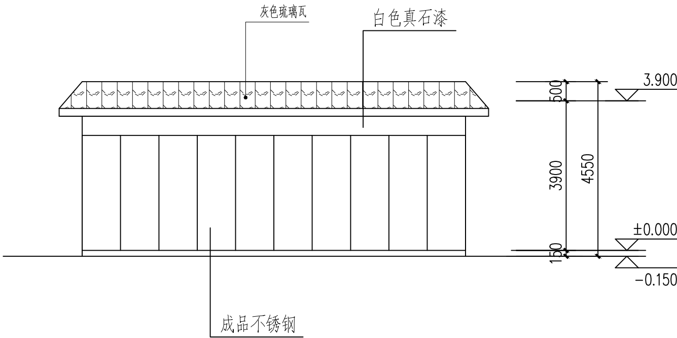
消防水池和水池泵侧立面图 1:100
