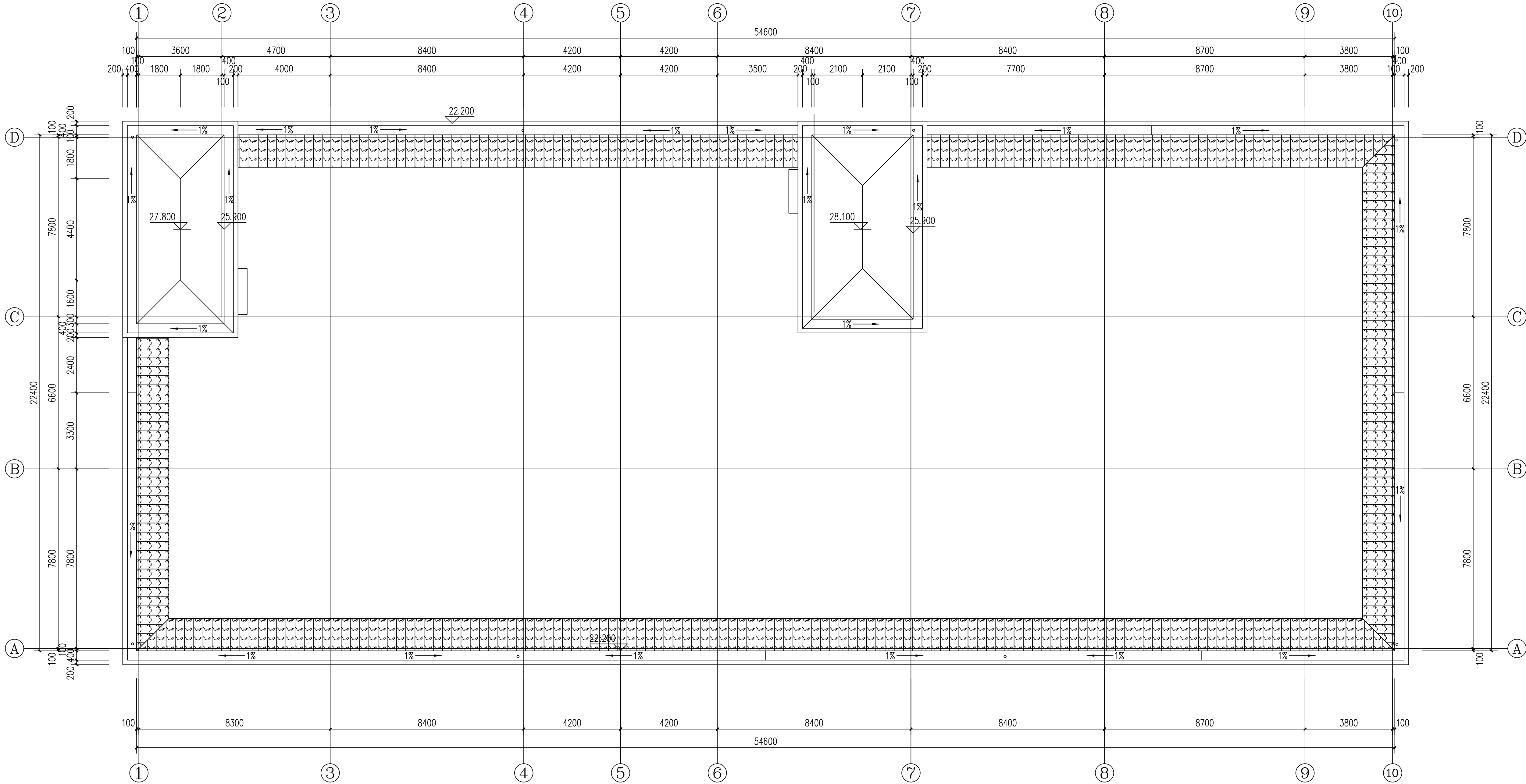
屋顶层平面图 1:100
