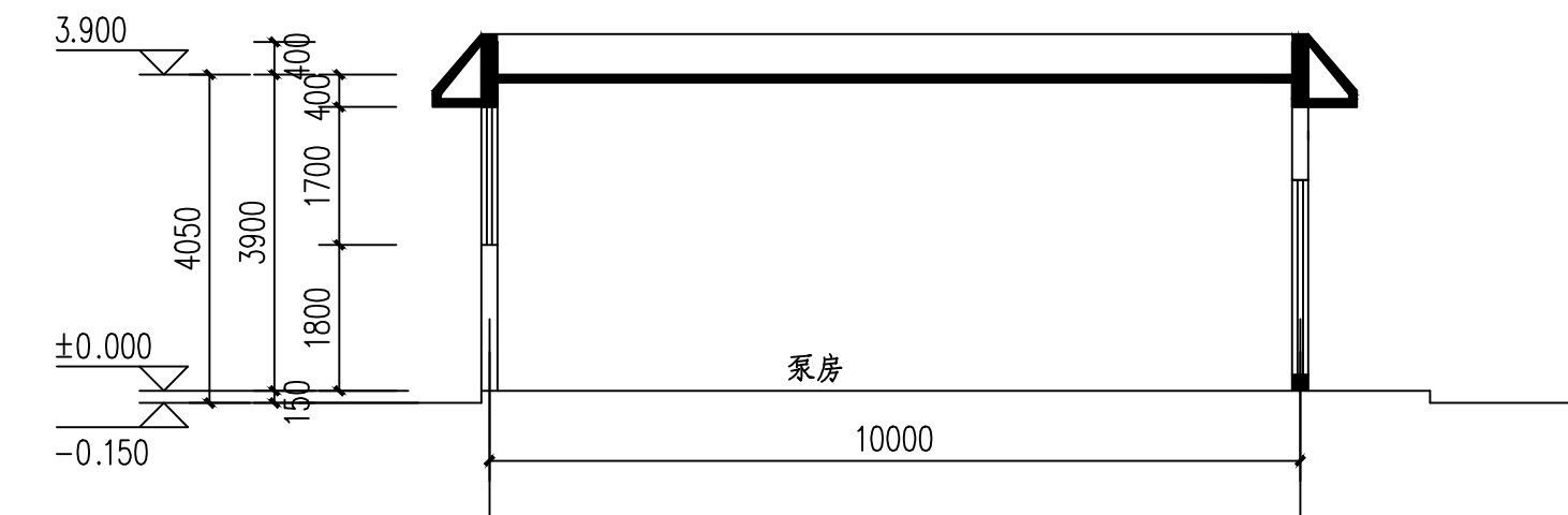
1-1剖面图 1:100
