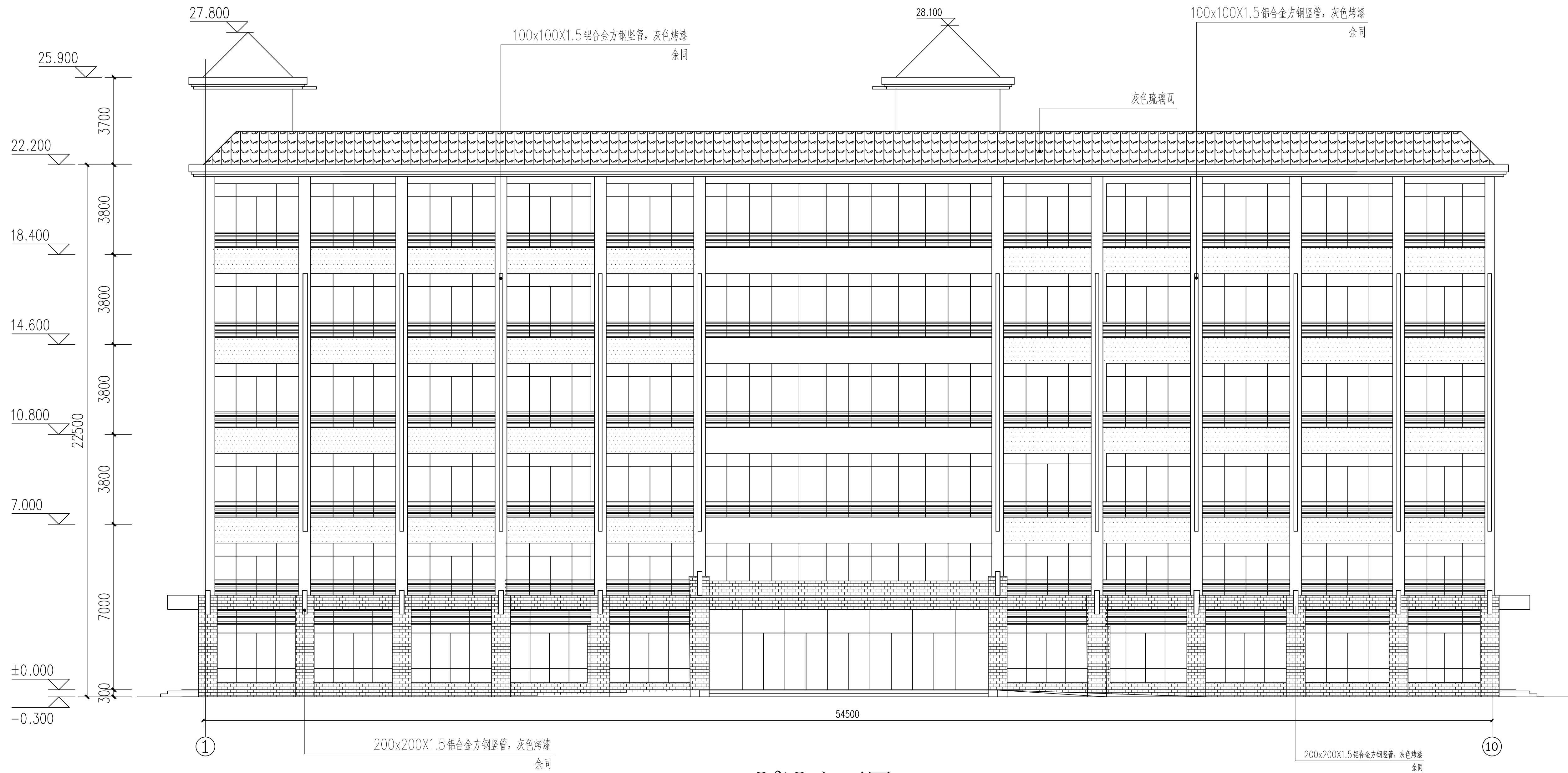
①~⑩立面图 1:100
