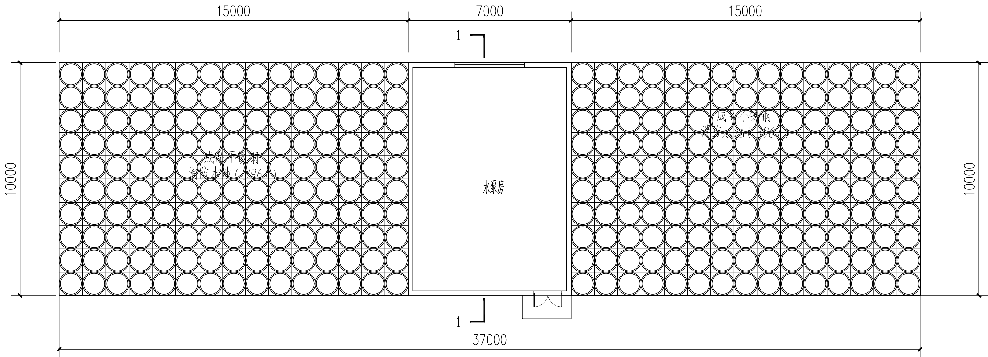
消防水池和水池泵一层平面图 1:100 本层建筑面积：70平米
