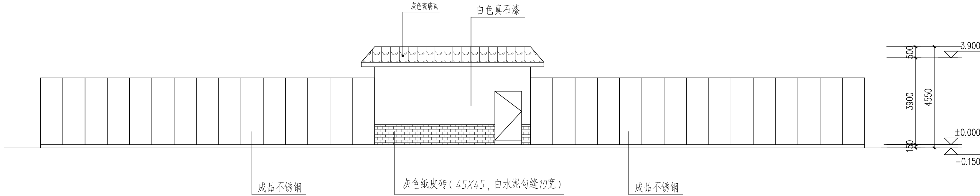
消防水池和水池泵正立面图 1:100
