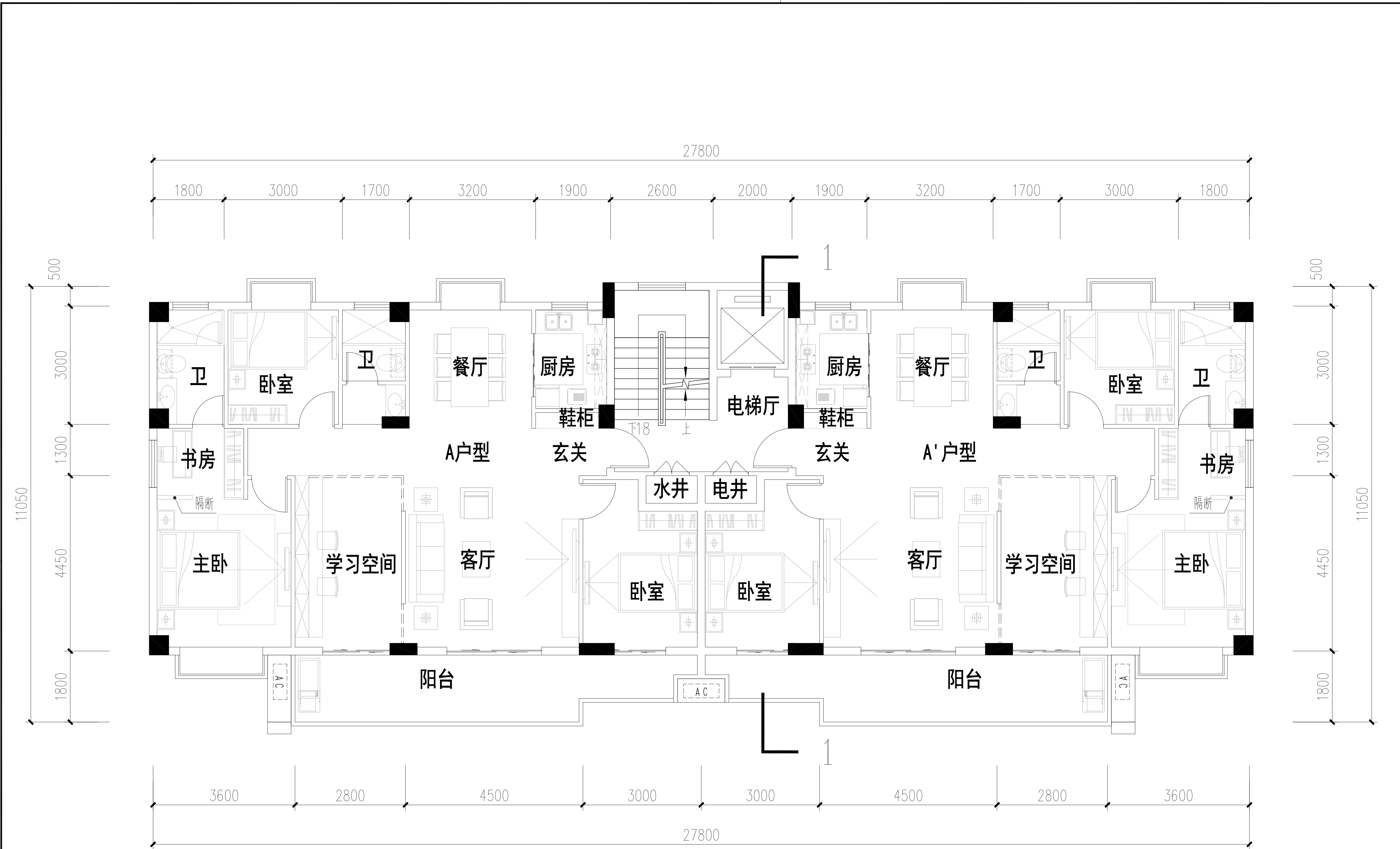
F地块 5#, 6#, 7#, 8#, 9#, 10#, 15#, 18#, 19# 标准层平面图 1:150
