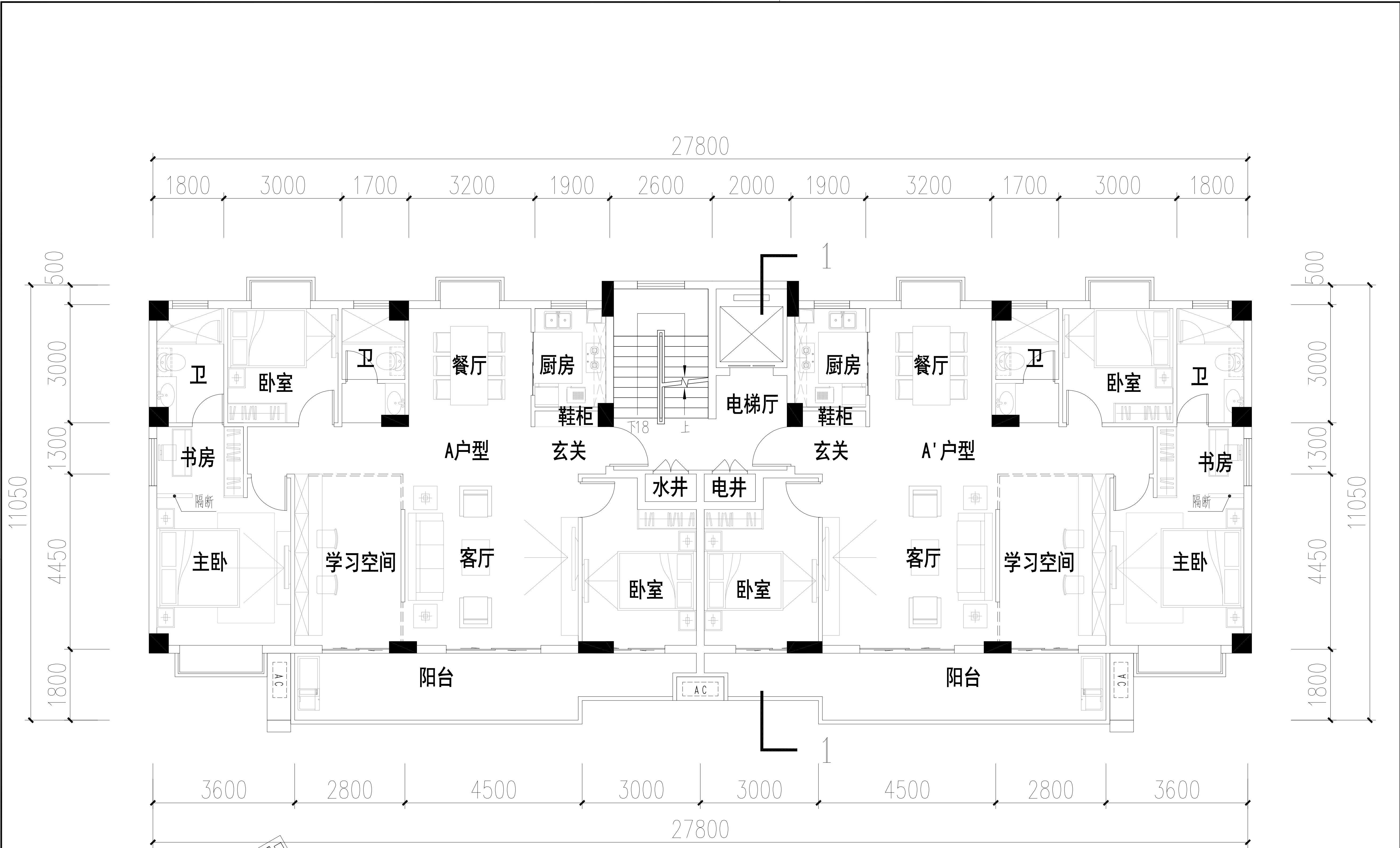
E地块27#标准层平面图 1:150
