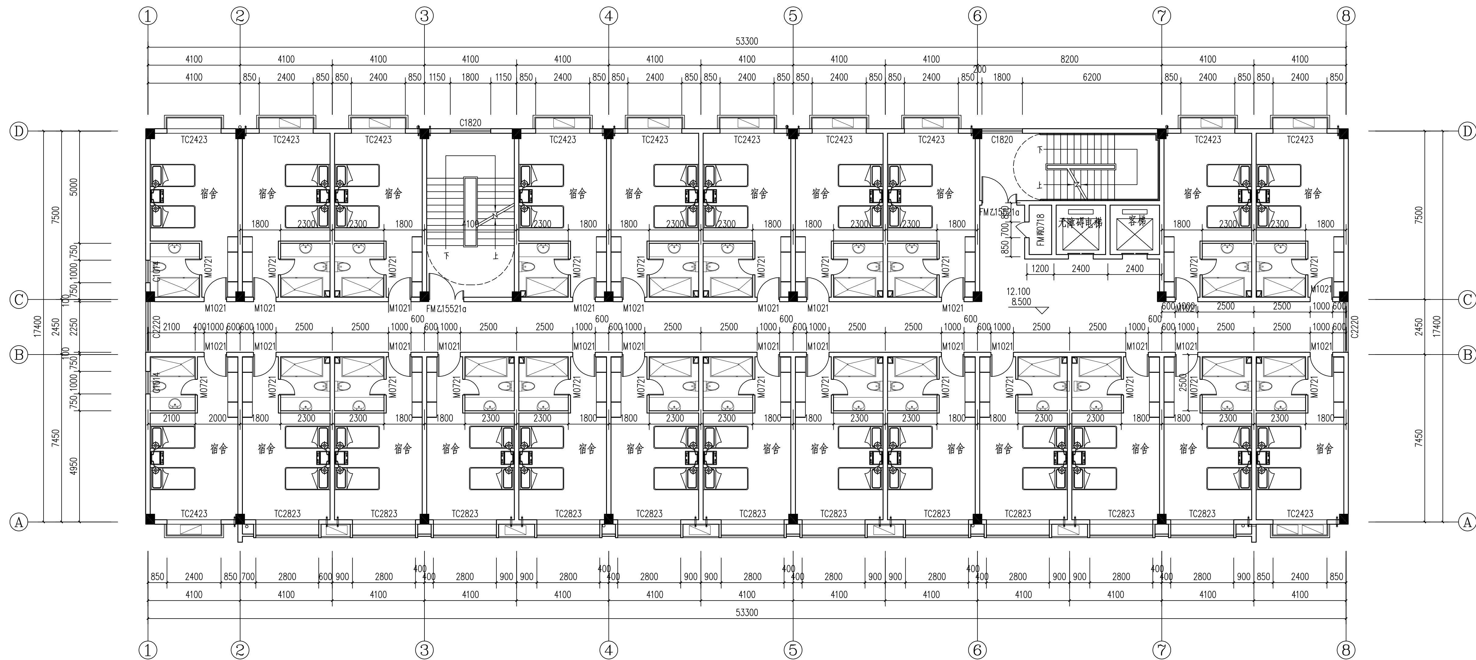
三~四层平面图 1:100
