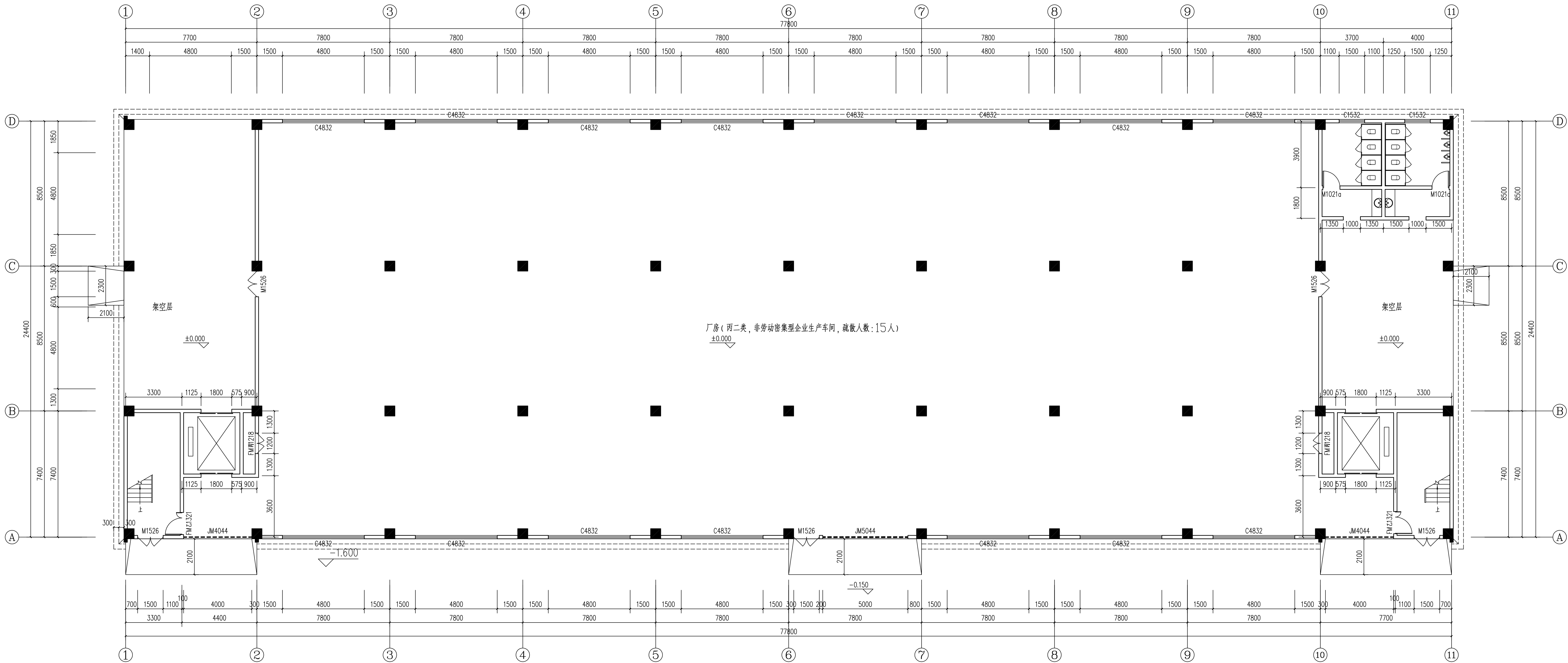
一层平面图 1:100
