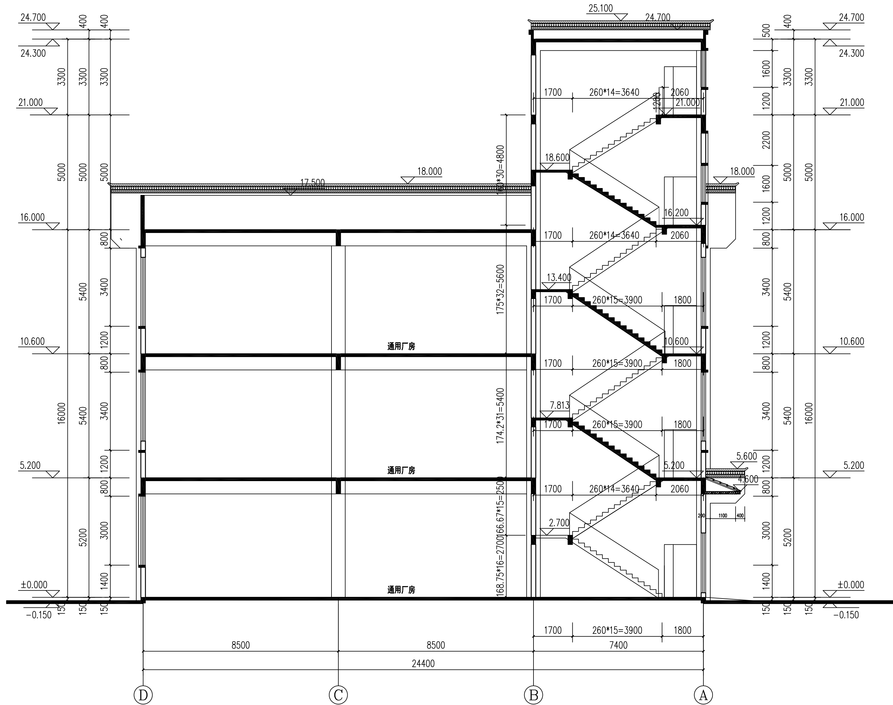
1-1剖面图 1:100
