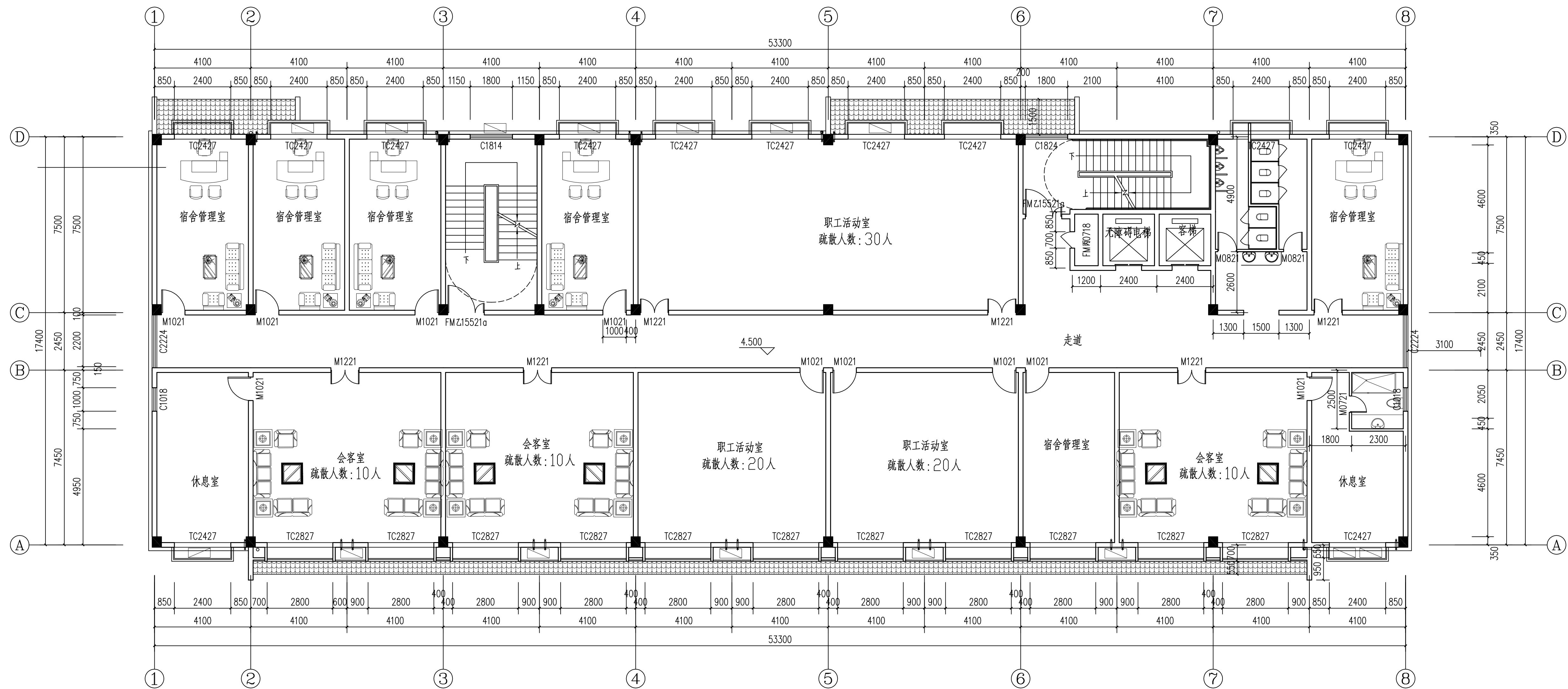
二层平面图 1:100
