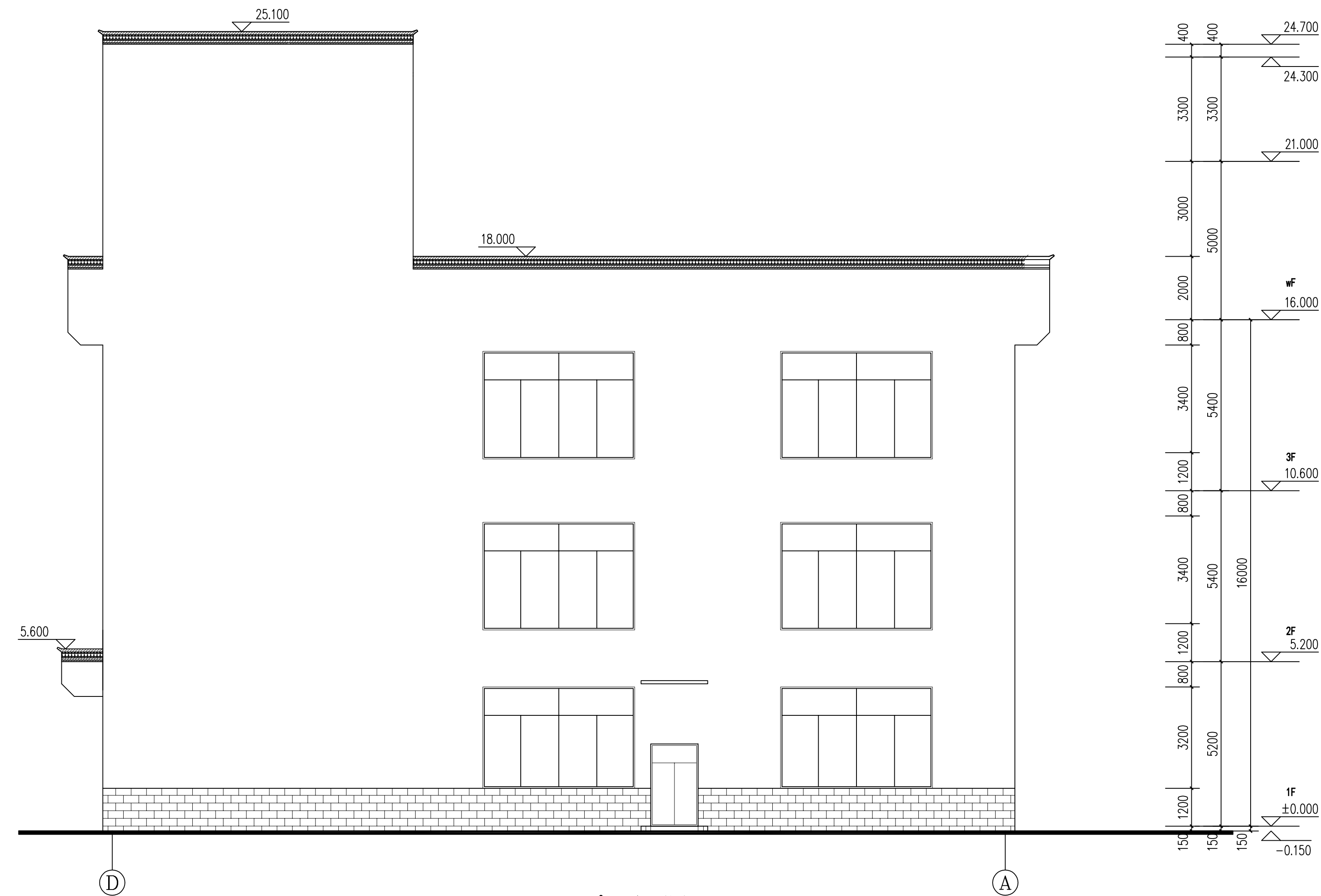
④~①立面图 1:100
