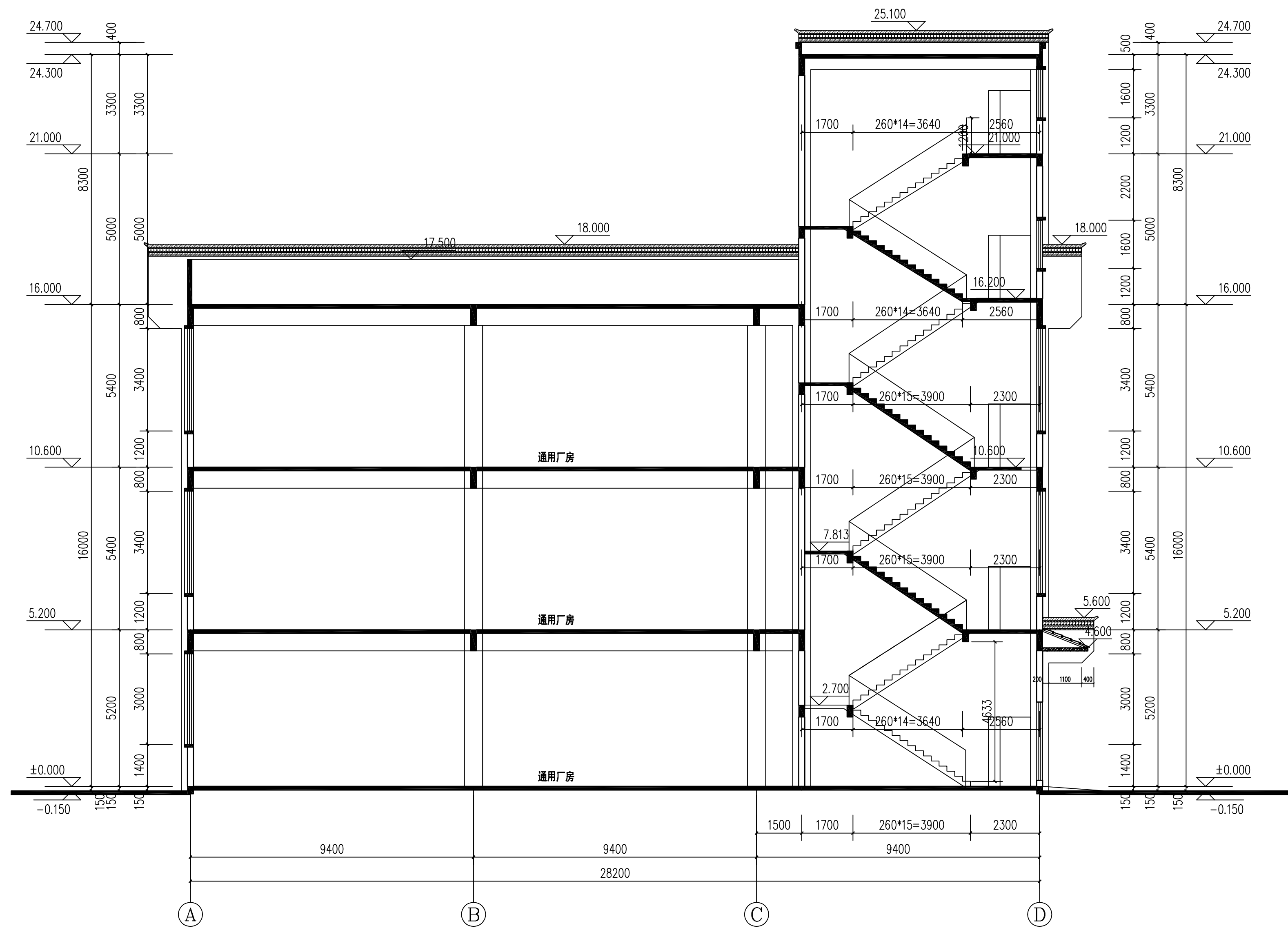
4#厂房1-1剖面图 1:100
