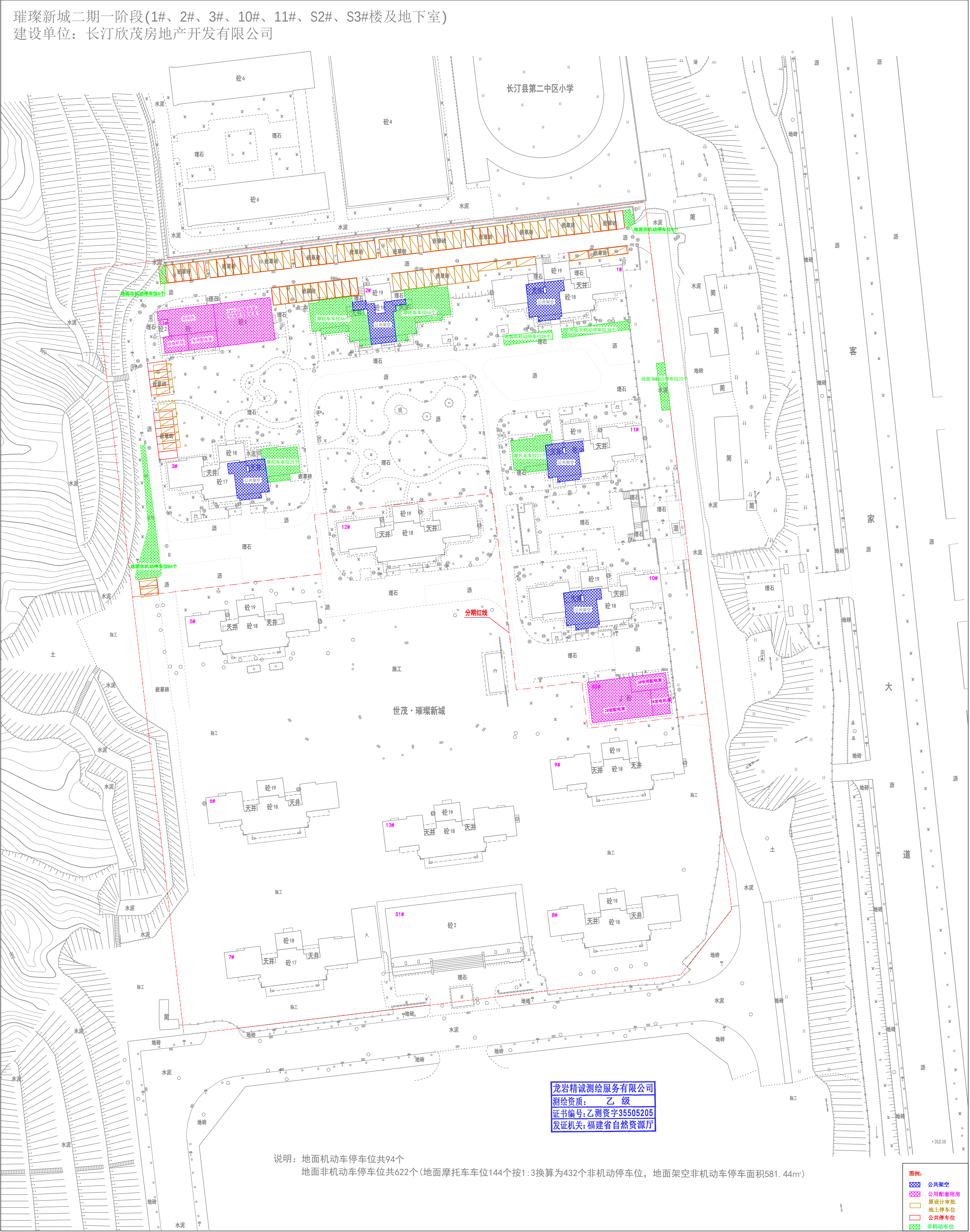
附件3：璀璨新城二期一阶段(1#、2#、3#、10#、11#、S2#、S3#楼及地下室)地上公共配套示意图
